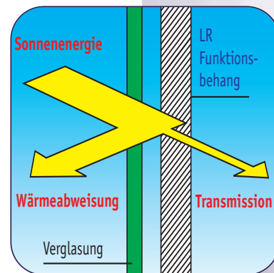
Funktionsschema der LR-Lamelle
